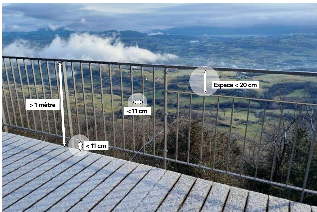
Dimensions du garde-corps installé sur le belvédère du sentier des Belvédères, (forêt domaniale de Clergeon) - ©A. Guézou (ONF)
