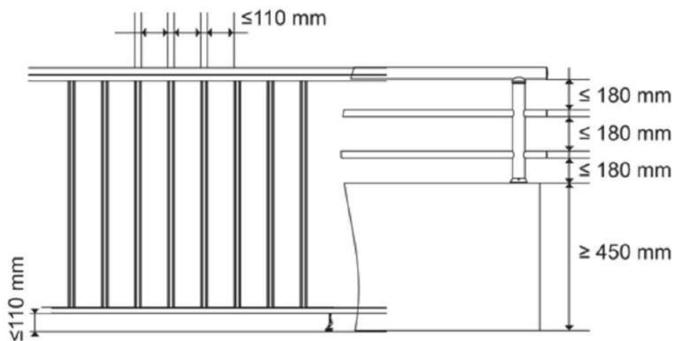
Dimensions d'un garde-corps selon la norme NF P 01-012
